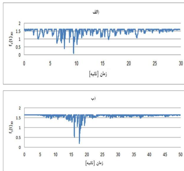
شکل ۱۲. قسمتی از تاریخچه زمانی ضریب اطمینان دینامیکی در نظر گرفته شده برای محاسبه \bar{f} با اعمال زلزله الف) طبس و ب) چی‌چی
