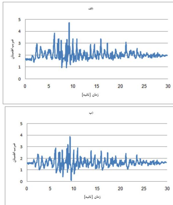
شکل ۱۰. تاریخچه زمانی ضریب اطمینان معادل تغییر مکان مجاز گوه در زلزله طیس مقیاس شده به 0.76g (الف) قبل از اعمال فیلتر بالاگذر (ب) پس از اعمال فیلتر بالاگذر
