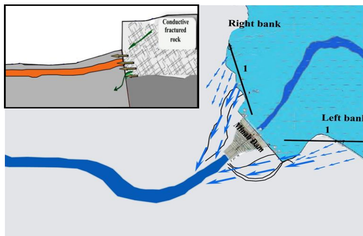
شکل ۱۵. طرح شماتیکی از نحوه قرارگیری سد و توده‌های سنگی در قطعه‌های ۱ از جناح چپ و قطعه ۶ از جناح راست
