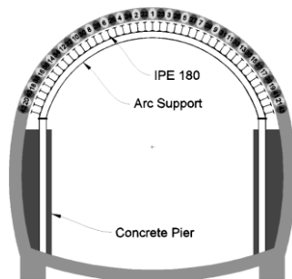
شکل ۱۲. مراحل تیر آهن رانی در تونل سبزه
