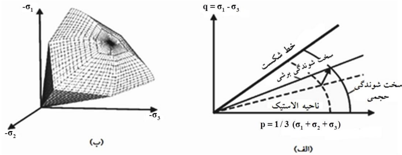
شکل ۶. سطح تسلیم برای مدل خاک سخت شونده در C=0 (الف) سخت شونده برشی و حجمی در فضای p-q (ب). سطح تسلیم کل در فضای تنش‌های اصلی [۳۱]
