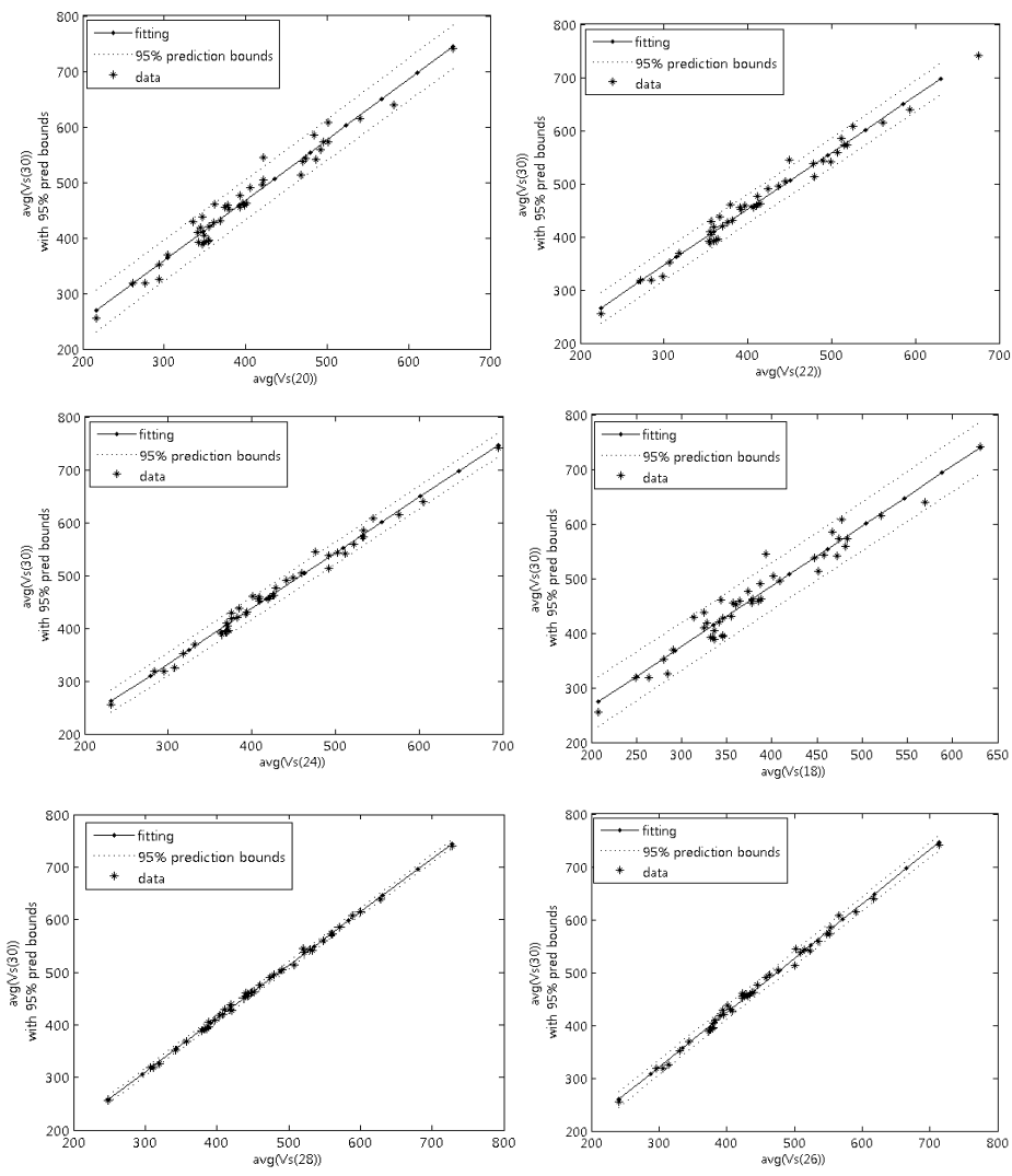
ادامه شکل ۷
