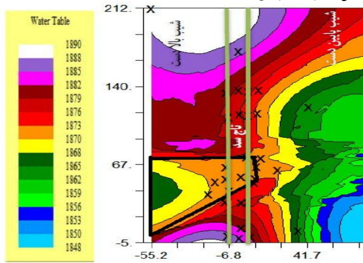
شکل ۵. نقشه دو بعدی هم تراز پیزومتری در بدنه سد جدول ۳. سطح ایستابی آب در پیزومترها نسبت به دریا
