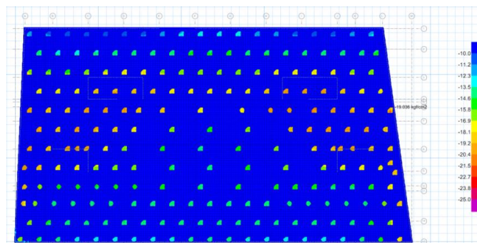
شکل ۵ پلان جانمایی و تنش‌های وارد بر ستون‌های بت‌گروت در طرح اولیه ( \text{kg/cm}^2 )
