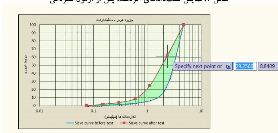
شکل ۸. نمایش محاسبه سطح بین دو نمودار دانه‌بندی قبل و بعد از فشرده‌گی
