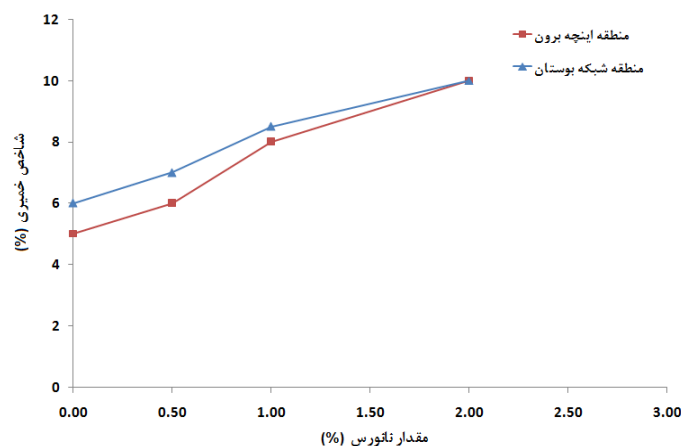
شکل ۱۳. تأثیر نوع خاک بر شاخص خمیری نمونه‌ها ناشی از افزودن نانوسیس
