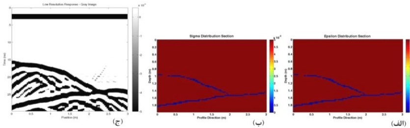
شکل ۶. الف) مقطع توزیع گذردهی دی‌الکتریک، ب) مقطع توزیع هدایت الکتریکی و ج) پاسخ GPR مدل منشور دوبعدی گرانیته شامل دو ناپوستگی متقاطع
