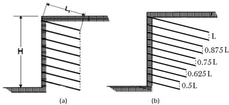
شکل ۵. چیدمان مختلف طول میخ‌ها
