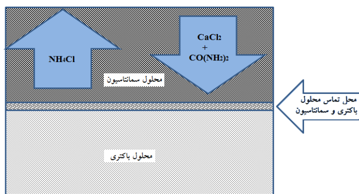
شکل ۷. نحوه ایجاد جریان همرفتی در محلول سمنتاسیون درون نمونه خاک
