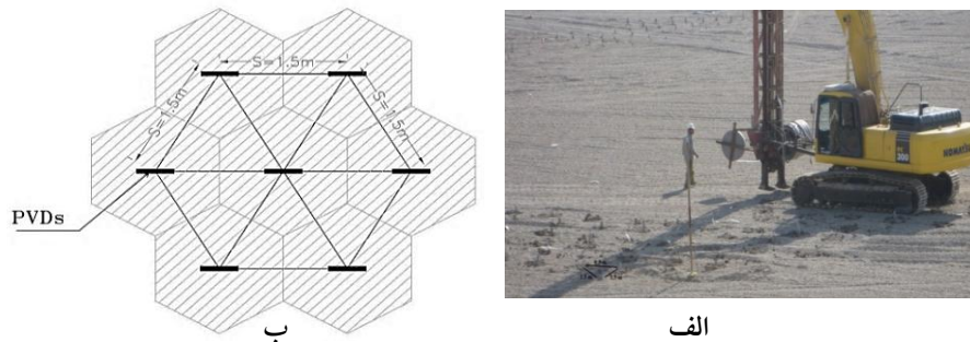
شکل ۶. الف) نمایی از اجرای زهکش‌های نواری در زیر خاکریزها ب) آرایش زهکش‌ها در پلان
