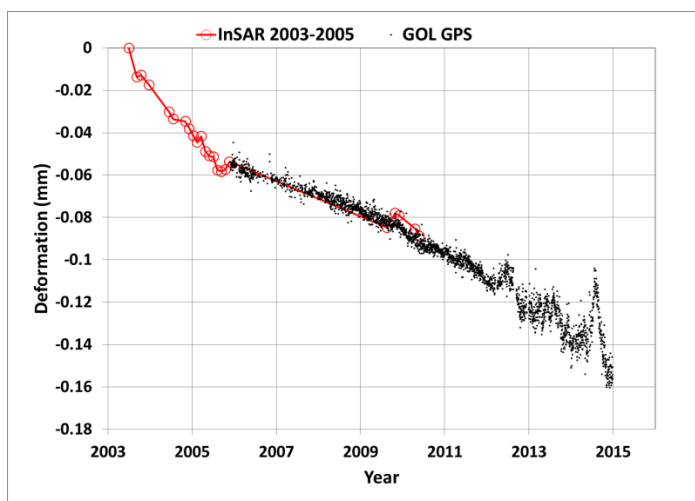
شکل ۱۱. ج) مقایسه مشاهدات پیوسته ایستگاه دائم ژئودینامیک GOL با نتایج حاصل از تداخل‌سنجی راداری
