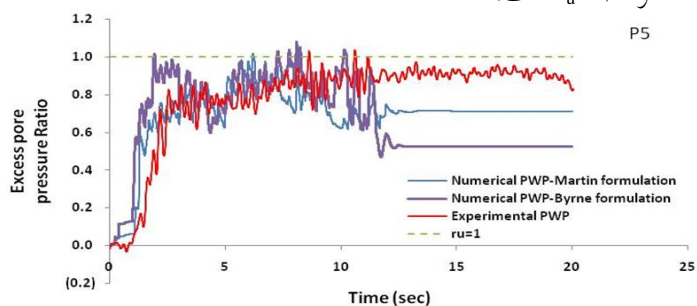
شکل ۱۱. مقایسه تاریخچه نسبت فشار آب حفره‌ای مدل‌سازی عددی و آزمایش سانتی‌فوتژ در عمق ۱/۴۵ متر
