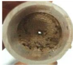
تغییر قطر سوراخ در پایان آزمایش در نمونه خاک منطقه بق قجه بالا یا دانسته حداکثر
