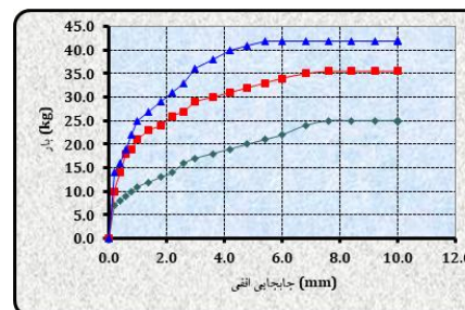
شکل ۷. نمودار بار-جایجایی افقی (خاک تثبیت شده با ۱٪ آهک و ۵٪ سرباره)
