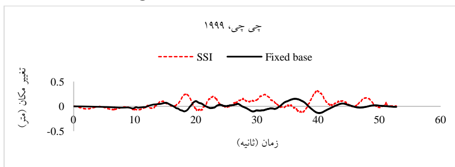
شکل ۵. تغییر مکان جانبی نسبی عرشه پل نسبت به کلاهک با در نظرگیری و بدون در نظرگیری اثر اندرکنش خاک-سازه تحت اثر زلزله چی چی ۱۹۹۹
