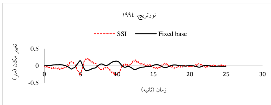
شکل ۴. تغییر مکان جانبی نسبی عرشه پل نسبت به کلاهک با در نظرگیری و بدون در نظرگیری اثر اندرکنش خاک-سازه تحت اثر زلزله نورتریج ۱۹۹۴
