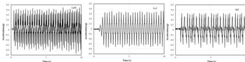
شکل ۵. نمونه‌ای از تاریخچه‌های زمانی شتاب در فرکانس ۳ هرتز و شتاب ورودی ۰/۳g در شتاب‌سنج A_2 تحت بارگذاری الف) مستطیلی، ب) سینوسی و ج) مثلثی
