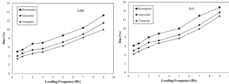
شکل ۲۴. تغییرات میانگین نسبت میرایی ( D_m ) با فرکانس بارگذاری در شتاب ورودی الف) 0.1g ، ب) 0.3g
