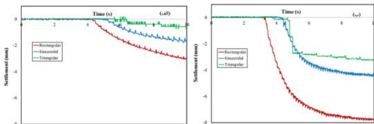
شکل ۶. الف. نمونه‌ای از تاریخچه‌های زمانی جابجایی قائم در فرکانس ۳ هرتز و شتاب ورودی الف) 0.1g ، ب) 0.1/8g
