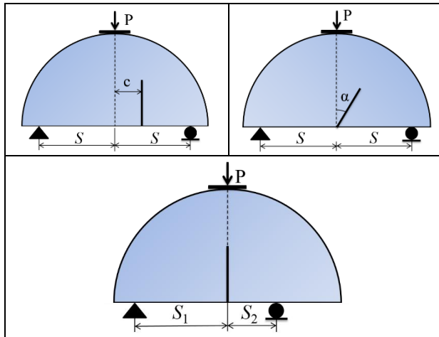
شکل ۲. حالت‌های مربوط به بارگذاری مود ترکیبی I/II جدول ۱. اندازه‌های آزمایش و شرایط بارگذاری مربوط
