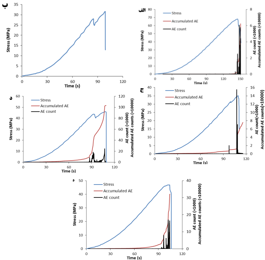
شکل ۵. نمودار تنش و AE در برابر زمان برای نمونه‌های مختلف الف (S2، ب) S-0-2، ج) S-30-5، د) S-60-5، ه) S-90-3
