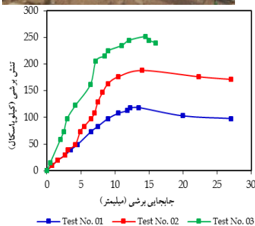
شکل ۱۰. آزمایش برش برجا (بالا) و نمودار تنش- جابه جایی برشی (پایین)
