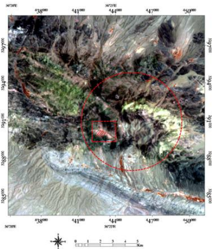
شکل ۳. آلتراسیون‌های آرژلیک و فلیک به‌رنگ صورتی تا قرمز (مربع قرمز) آلتراسیون پروپلیتیک به‌رنگ سبز
