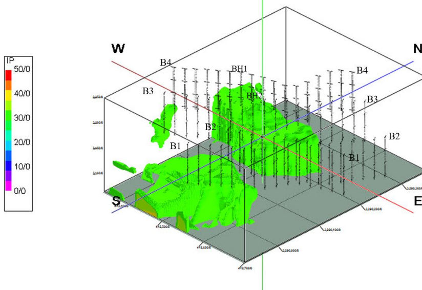
شکل ۱۴. الف) نمایش سه بعدی پلازاسیون القایی، ب) نمایش سه بعدی پلازاسیون القایی با مقادیر بیش‌تر از ۳۸ms
