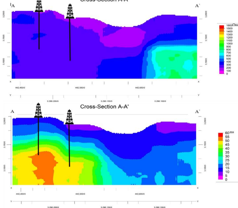
شکل ۱۳. مقطع مقاومت ویژه و پلاریزاسیون‌القایی یروفیل AA' ایجاد شده به وسیله نرم‌افزار RockWork
