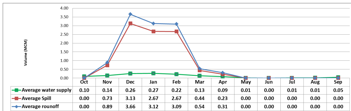
شکل ۱۳. میانگین ماهانه حجم رواناب، سرریز و حجم کل تأمین آب سد سنا بر حسب میلیون متر مکعب
