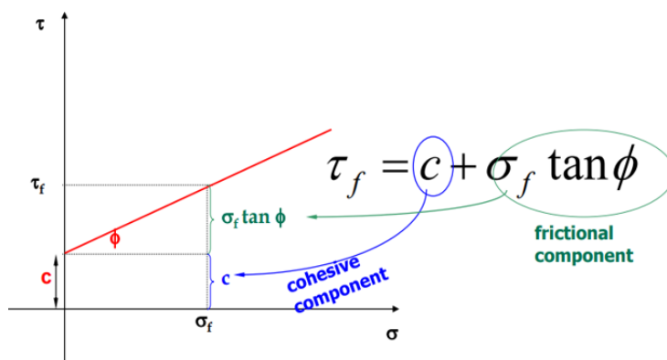
شکل ۵. نمودار بدست آمده از آزمایش مقاومت برشی مستقیم و مقادیر c و \phi (Smith and Sachan, 2015) Fig. 5. Graph obtained from direct shear strength test and values of c and \phi (Smith and Sachan, 2015)
