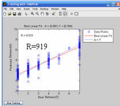
نتایج آموزش شبکه پیش‌بینی رفتار آب‌گذری یا استفاده از ۶ پارامتر
