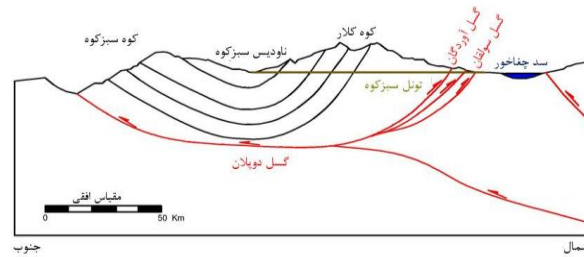
شکل ۳. مقطع ناودیس سبزکوه از سد چغاقور تا محدوده گسل دویلان [۱۷]
