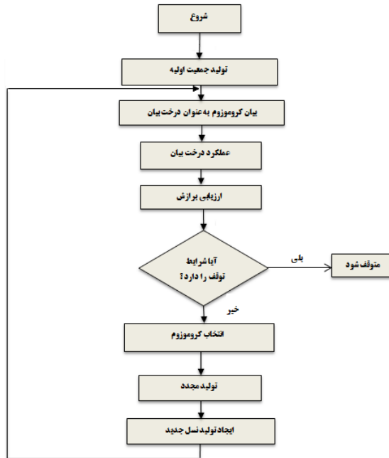
شکل ۲. الگوریتم جپ [۲۵]
