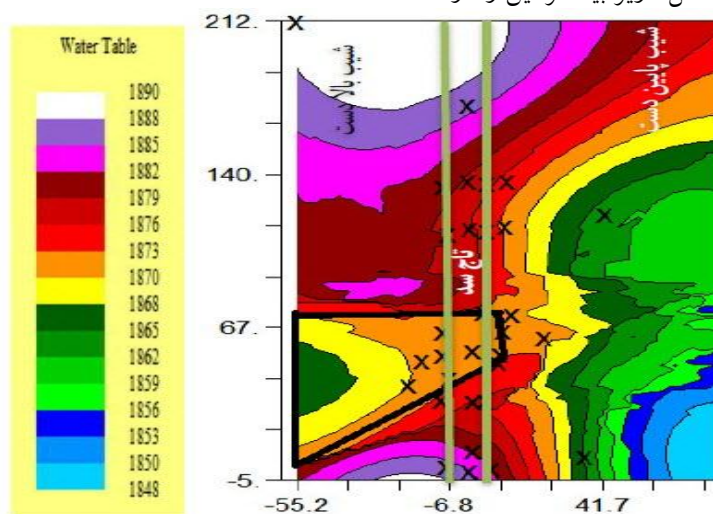
شکل ۵. نقشه دو بعدی هم تراز پیژومتریک در بدنه سد جدول ۳. سطح ایستابی آب در پیژومترها نسبت به دریا
