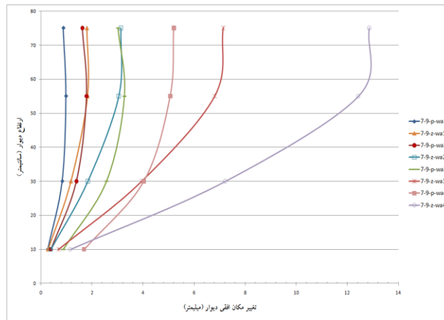
شکل ۸. تأثیر نحوه‌ی اجرای تسمه‌های پلیمری بر تغییر مکان دیوار
