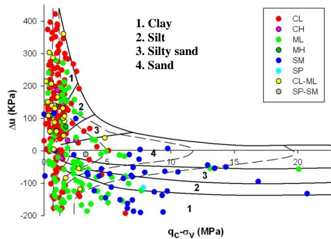
شکل ۳. طبقه‌بندی خاک با استفاده از روش جونز و راست [۷] و مقایسه آن با نتایج آزمایش دانه‌بندی در تحقیق حاضر
