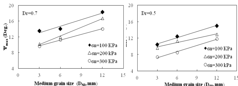
شکل ۶. تغییرات زاویه اتساع حداکثر در خاک‌های مختلف برای تراکم نسبی الف) ۵۰ درصد، ب)
