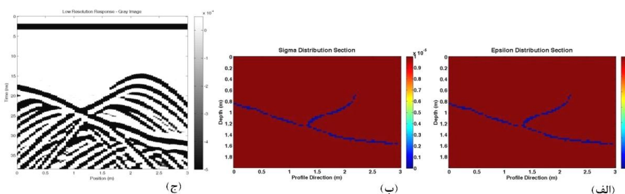
شکل ۸. الف) مقطع توزیع گذردهی دی‌الکتریک، ب) مقطع توزیع هدایت الکتریکی و ج) پاسخ GPR یک مدل منشور دوبعدی از جنس مرم‌مر شامل دو ناپیوستگی متقاطع
