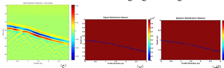
شکل ۷. الف) مقطع توزیع گذردهی دی‌الکتریک، ب) مقطع توزیع هدایت الکتریکی و ج) پاسخ GPR مدل منشور دوبعدی از جنس مرم‌مر شامل یک ناپیوستگی سرتاسری
