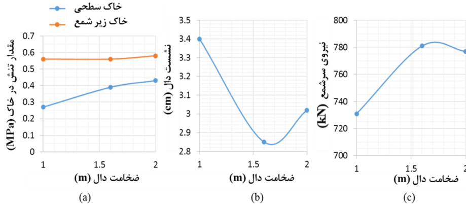
شکل ۹. اثر تغییر ضخامت دال در a . تنش در خاک، b . نشست دال و c . نیروی سر شمع
