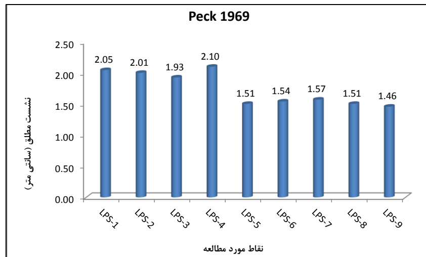
شکل ۵. نمودار ستونی نشست‌های پیش‌بینی شده در مسیر تونل ابوذر [۱]
