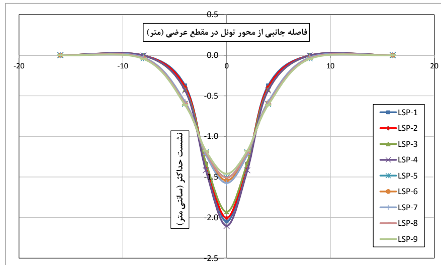
شکل ۶. منحنی‌های گودی نشست (پیش‌بینی شده) در مقاطع عرضی برای نقاط بررسی شده [۱] جدول ۷. ارزیابی نشست به روش تحلیلی لگاناتان و پولوس [۲۲] با فرض g=0.19 \text{ m} و
