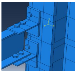
شکل ۸. اتصال سپری (g)
