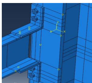
شکل ۵. اتصال نبشی نشیمن ساده جوشی (f)
