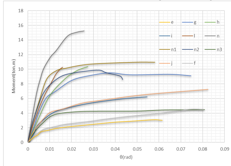
شکل ۲۵. پوش منحنی لنگر - چرخش نمونه‌ها تحت بارگذاری چرخه‌ای
