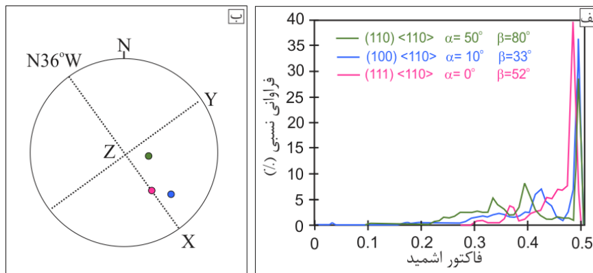
شکل ۶. نتایج تجزیه عامل اشمید، الف) منحنی‌های فراوانی عامل اشمید برای سه سیستم لغزشی موجود در بلورهای هالیت، ب) موقعیت تنش‌های تراکمی مربوط به بیش‌ترین مقدار عامل اشمید برای هر سیستم لغزشی در استریوت
