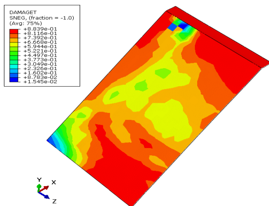
شکل ۱۰. مقایسه خرابی روکش بتنی تحت زلزله طیس در سه حالت؛ الف) خالی، ب) نیمه پر و ج) پر
