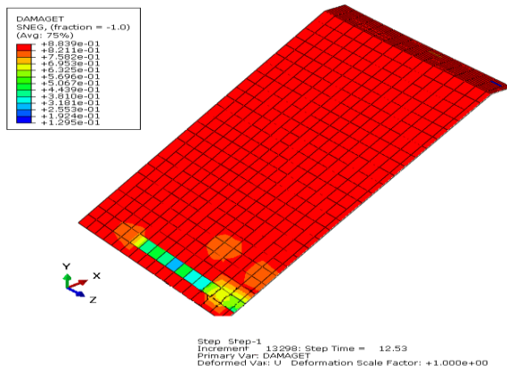
شکل ۷. مقایسه خرابی کششی روکش بتنی در سه حالت؛ الف) ضریب اصطکاک ۰/۵، ب) ضریب اصطکاک ۰/۷، ج) حالت مقید
