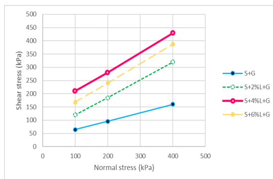
شکل ۹. پوش گسیختگی خاک تثبیت شده با درصدهای مختلف آهک و مسلح شده با ژئوگرید 4 \times 4 میلی‌متر بدون المان‌های متقاطع عرضی در درصد رطوبت بیش‌تر از بهینه
