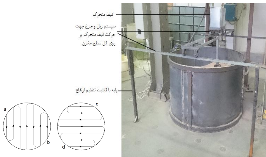
شکل ۵. الف) نمایی از سیستم هدایت قیف بر کل سطح مخزن ب) مسیر حرکت
