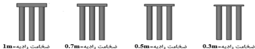
شکل ۷. حالت‌های آرایش پی رادیه-شمع با طول شمع‌های متغیر (واحد: متر)
