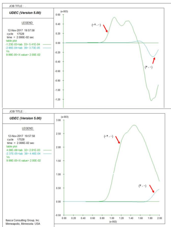
شکل ۱۰. تاریخچه زمانی الف) جابه‌جایی‌های افقی، ب) قائم در نقاط شاهد (۲، ۰) و (-۲، ۰) روی دیواره سمت چپ و راست رمپ در مدت زمان ۲۰ میلی‌ثانیه از اعمال بار دینامیکی
