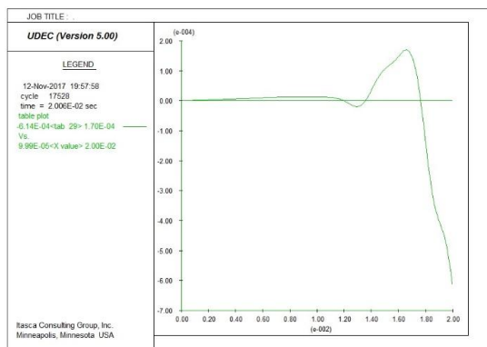
شکل ۹. تاریخچه زمانی جابه‌جایی‌های الف (افقی، ب) قائم در نقطه شاهد (۰، ۲/۱) روی سقف رمپ پس از گذشت مدت زمان ۲۰ میلی‌ثانیه از اعمال بار دینامیکی انفجار
