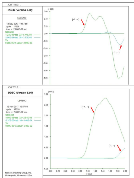
شکل ۱۰. تاریخچه زمانی الف) جابه‌جایی‌های افقی، ب) قائم در نقاط شاهد (۰، ۲) و (-۲، ۰) روی دیواره سمت چپ و راست رمپ در مدت زمان ۲۰ میلی‌ثانیه از اعمال بار دینامیکی
