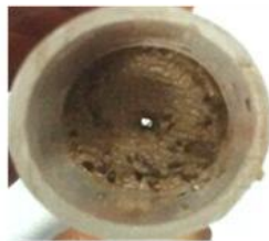
تغییر قطر سوراخ در پایان آزمایش در نمونه خاک منطقه بق قجه بالا با دانسیته حداکثر
