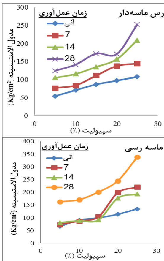
شکل ۳. تغییرات مدول الاستیسیته خاک‌های الف) ماسه رسی، ب) رس ماسه‌دار تثبیت شده با سیپولیت در درصد‌ها و زمان‌های عمل‌آوری متفاوت
