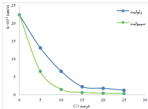
شکل ۶. نمودار تغییرات نفوذپذیری در درصدهای متفاوت زئولیت و سیولیت
