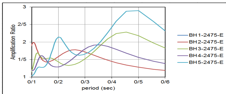
شکل ۱۴. طیف تقویت پروفیل‌های انتخابی با دوره بازگشت ۲۴۷۵ سال خروجی برنامه ارا
