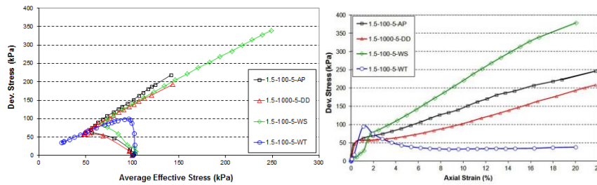
شکل ۴. نمودارهای تنش کرنش محوری ترکیبات شکل ۵. نمودارهای مسیر تنش ترکیبات ماسه و رس ماسه و رس (1.5-100-5-WT;DD;WS;AP) (1.5-100-5-WT;DD;WS;AP)
